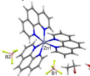
Fig. 1. Structure of [\text{Zn}(\text{phen})_3](\text{BF}_4)_2 \cdot \text{EtOH} \cdot \text{H}_2\text{O}
